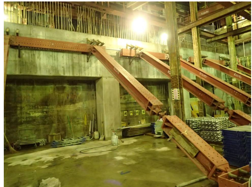
④地下広場(半蔵門線側) 平成27年4月 斜梁盛替
