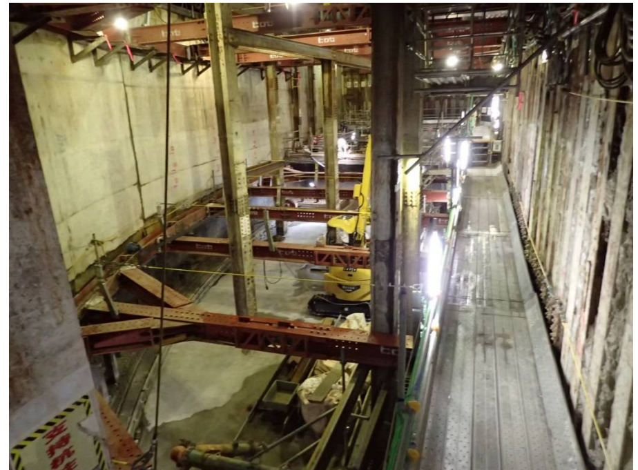
④東口地下広場 躯体構築状況(B2F)
